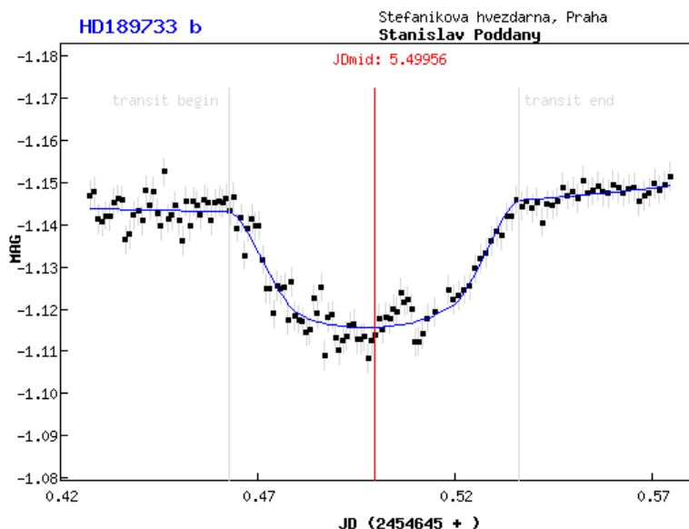
Obrázek 6: Výsledek fitovací procedury v on-line protokolu na zasílání pozorování tranzitů do databáze TRESKA. Modrá čára – modelová křivka, černé body jsou CCD pozorování.
